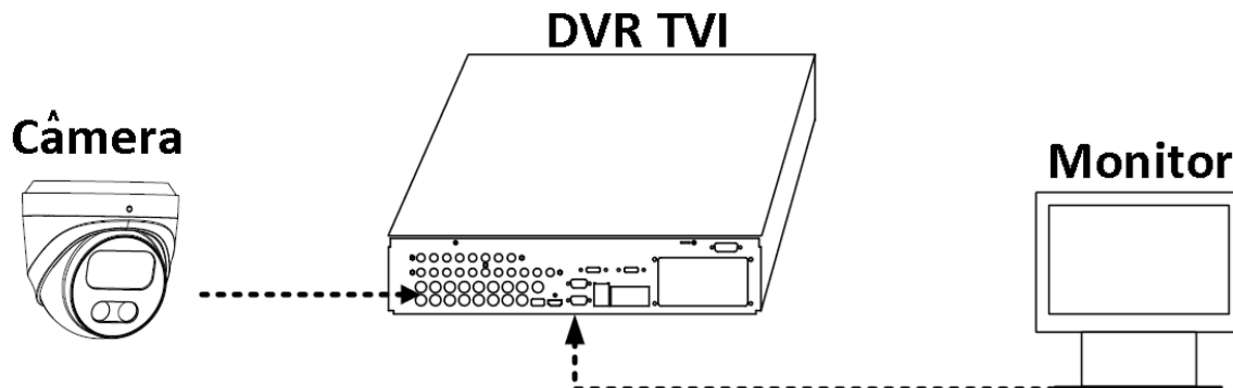
Figura 3.1: Conexão
