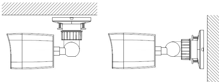
Figura 2.2 Parafuse a câmera ao teto ou a parede
