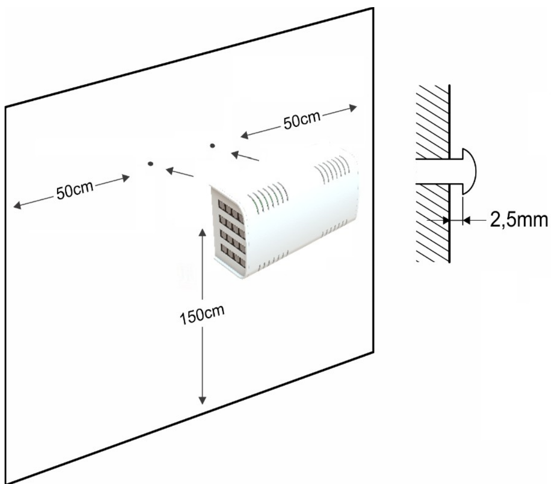
Figura 7: Fixação da central Optymus 66
