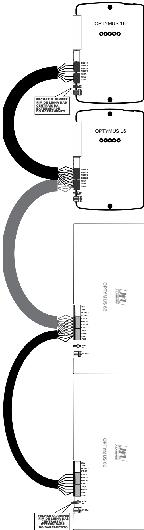
Figura 19: Esquema de interligação entre centrais Optymus 16 e Optymus 66
