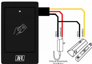
Fonte de Alimentação 12 à 28 Vc.c. Figura 6: Esquema de ligação do sensor de porta aberta.
