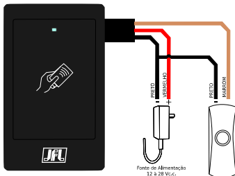
Fonte de Alimentação 12 à 28 Vc.c. Figura 5: Esquema de ligação botoeira.
