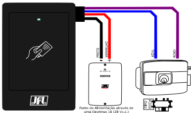
Figura 11: Esquema de ligação da fechadura eletromecânica com produto alimentado por uma Optymus 16.
